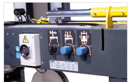
Hauptschalter jetzt in vertikaler Position, ergonomisches Bedienfeld
